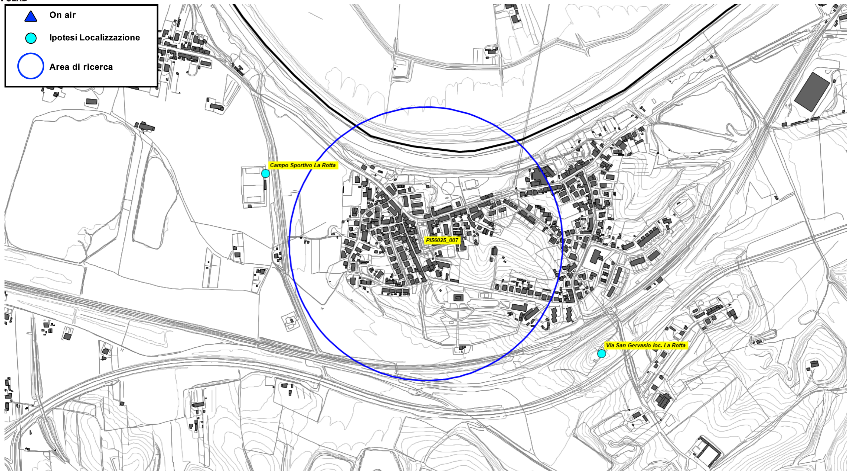
Fig. 30 Dettaglio piano di rete – gestore ILIAD
