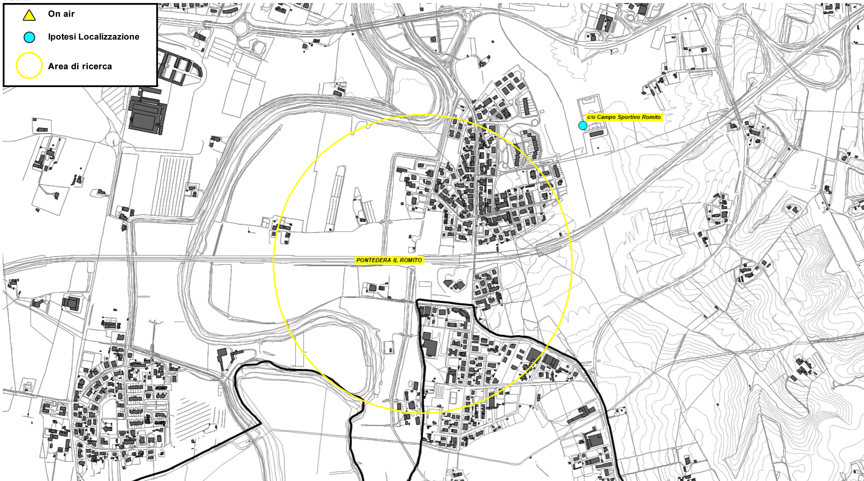
Fig. 25 Dettaglio piano di rete – Gestore WIND TRE
