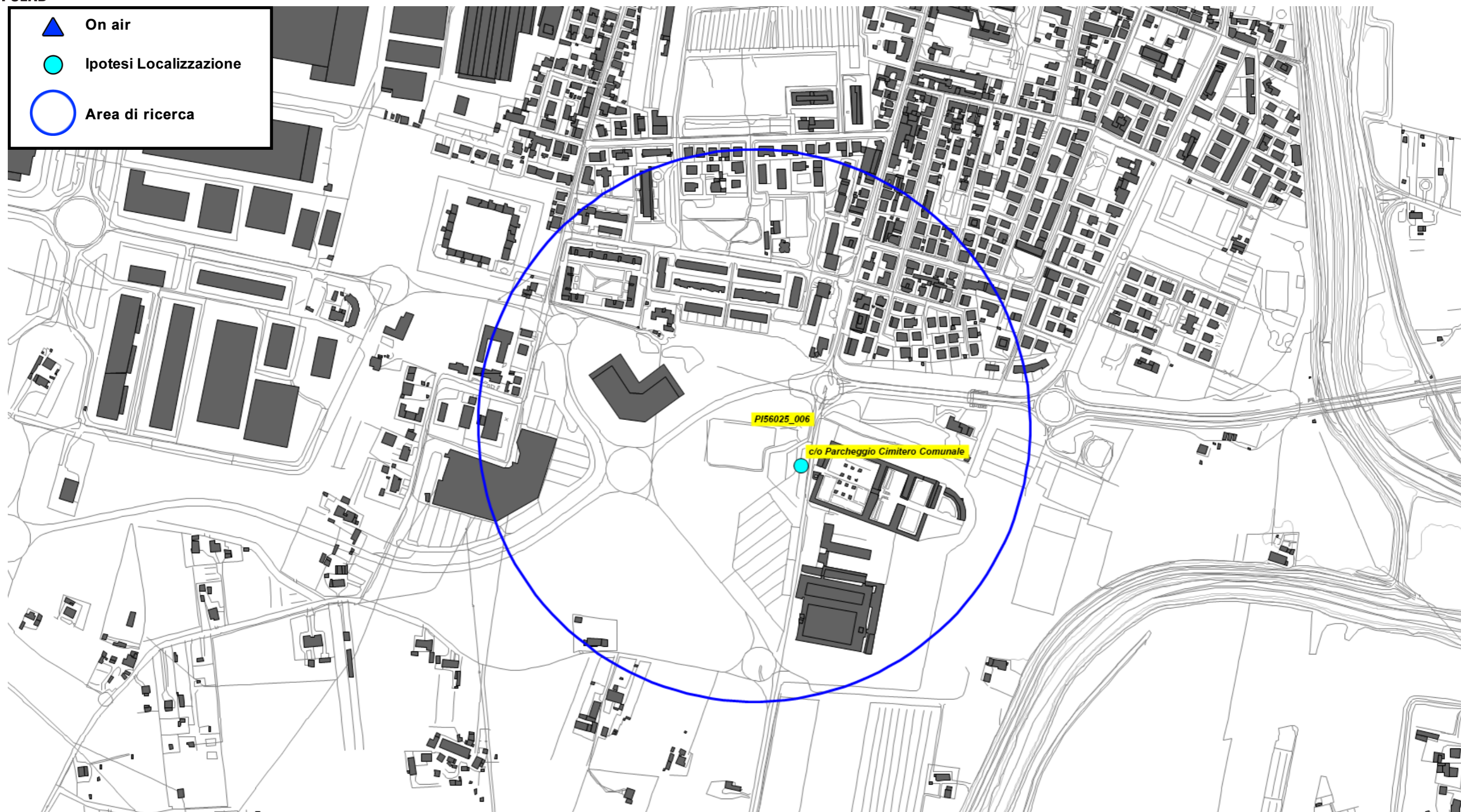
Fig. 28 Dettaglio piano di rete – gestore ILIAD
